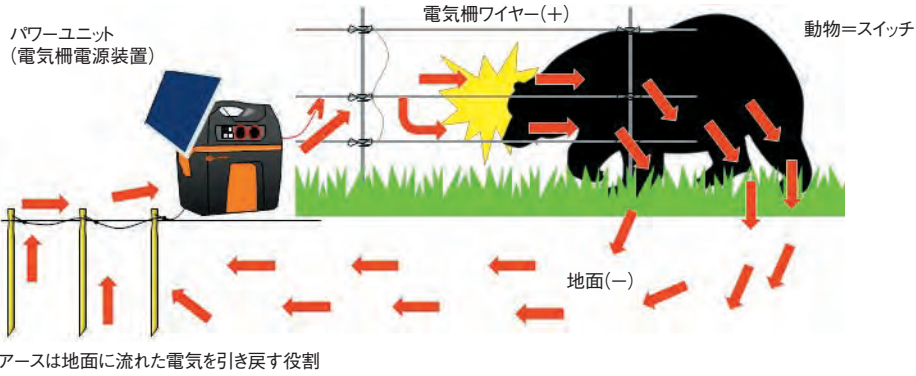
図11 正常な電気柵によりクマがショックを受けるしくみ （原図：サージミヤワキ(株)神武海氏提供）
